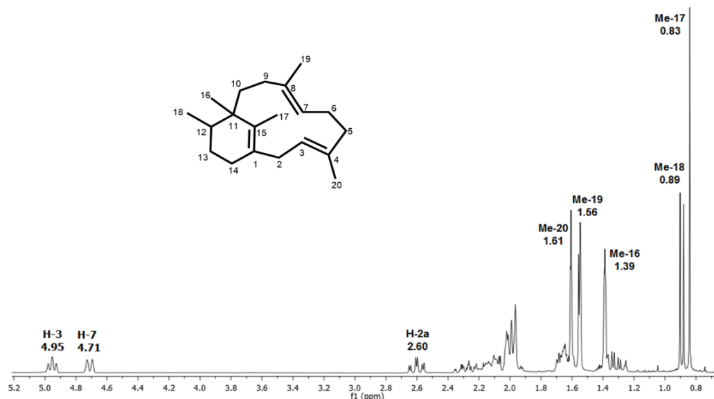
Figura 3. Espectro de NMR del fomacta-1(15),4,8-trieno tras purificación con sílica gel impregnada con \text{AgNO}_3 . Elaboración propia, espectro registrado en \text{CDCl}_3 y visualizado en MestReNova.
