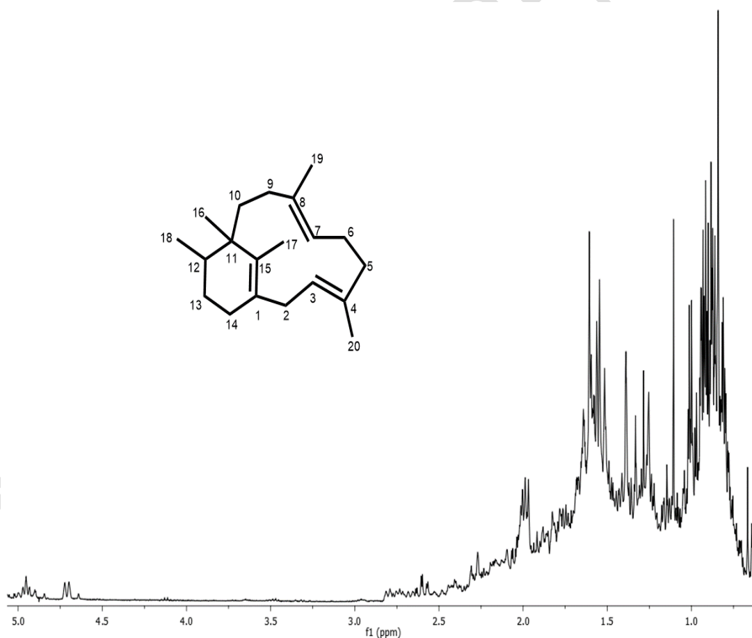
Figura 1. Espectro de NMR del crudo de reacción de verticilol con \text{BF}_3 . Elaboración propia, espectro registrado en \text{CDCl}_3 y visualizado en MestReNova .
