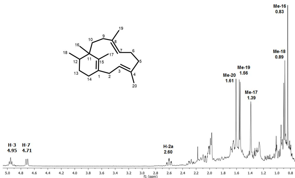
Figura 2. Espectro de NMR del fomacta-1(15),4,8-trieno tras purificación con sílica gel convencional. Elaboración propia, espectro registrado en \text{CDCl}_3 y visualizado en MestReNova.
